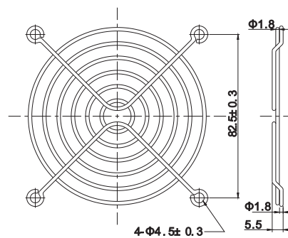
YM-09 ၏ 90mm အရွယ်အစား
