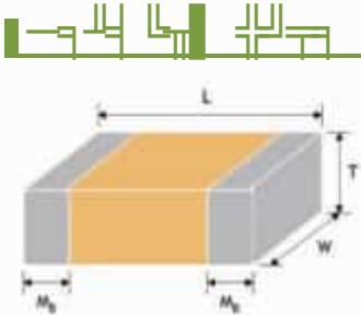
Рис. 1 контур MLCC
