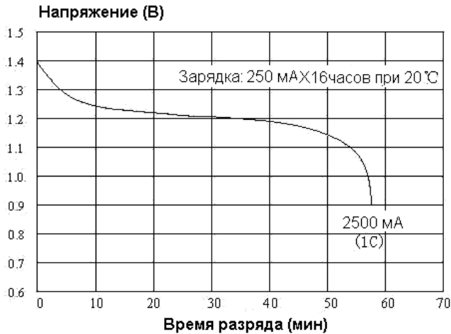
Высокая скорость разряда
