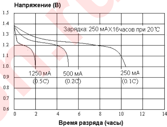
Низкая скорость разряда
