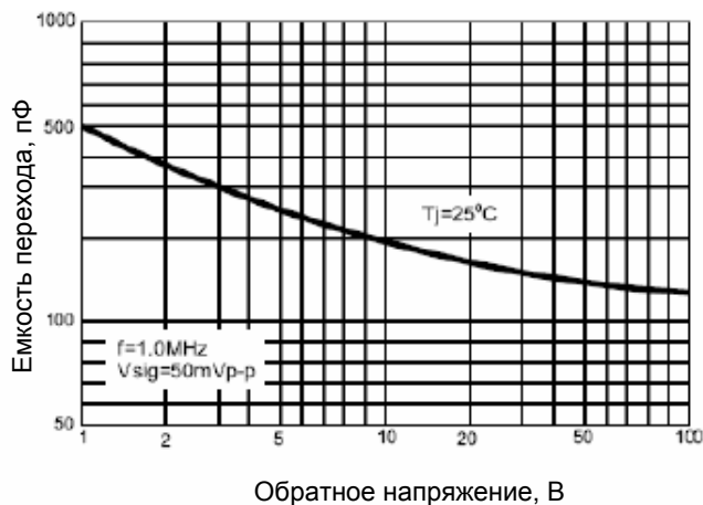
Рис. 5 – Типичная емкость перехода
