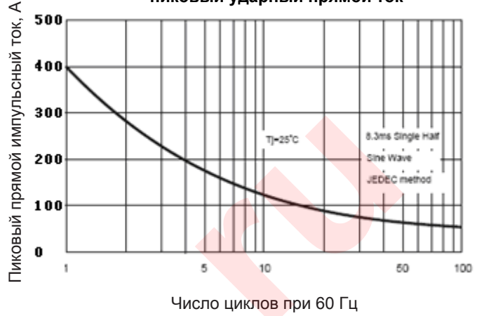
Рис.2- Максимальный неповторяющийся пиковый ударный прямой ток
