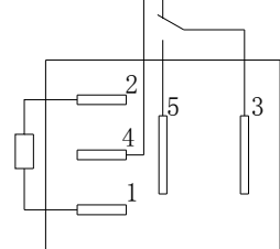
C 型接线图
