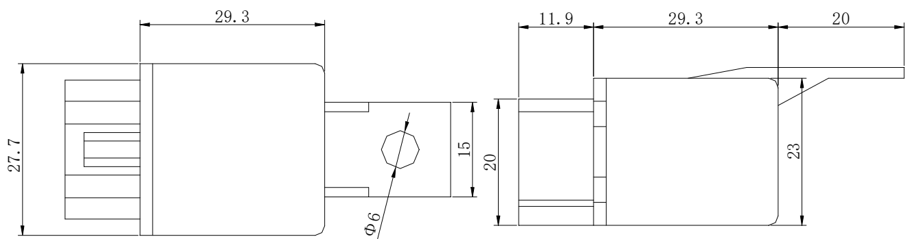
PC Board layout 安装图
