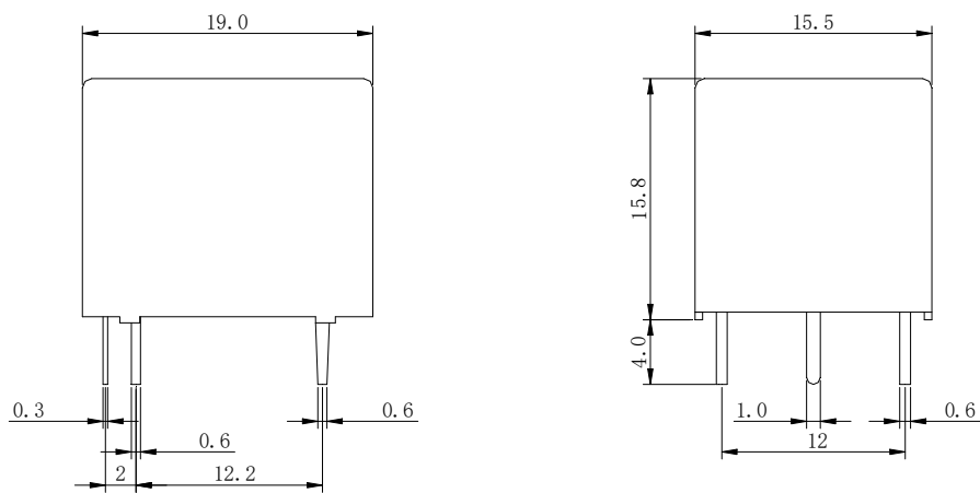
PC Board layout 安装图
