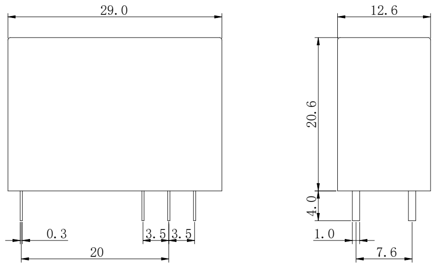
Outline Dimension 外形尺寸 (mm)
