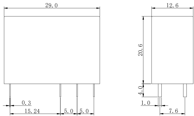
Outline Dimension 外形尺寸 (mm)
