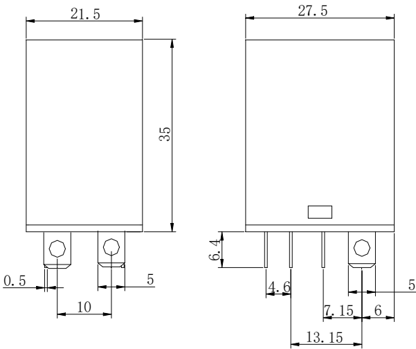
Wiring Diagram 接线图
