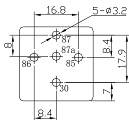
安装图（PCB）
