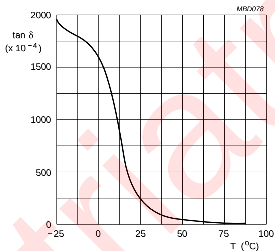
Рис. 5 Типичные изменения \tan \delta от температуры
