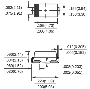
SMB(DO-214AA)
