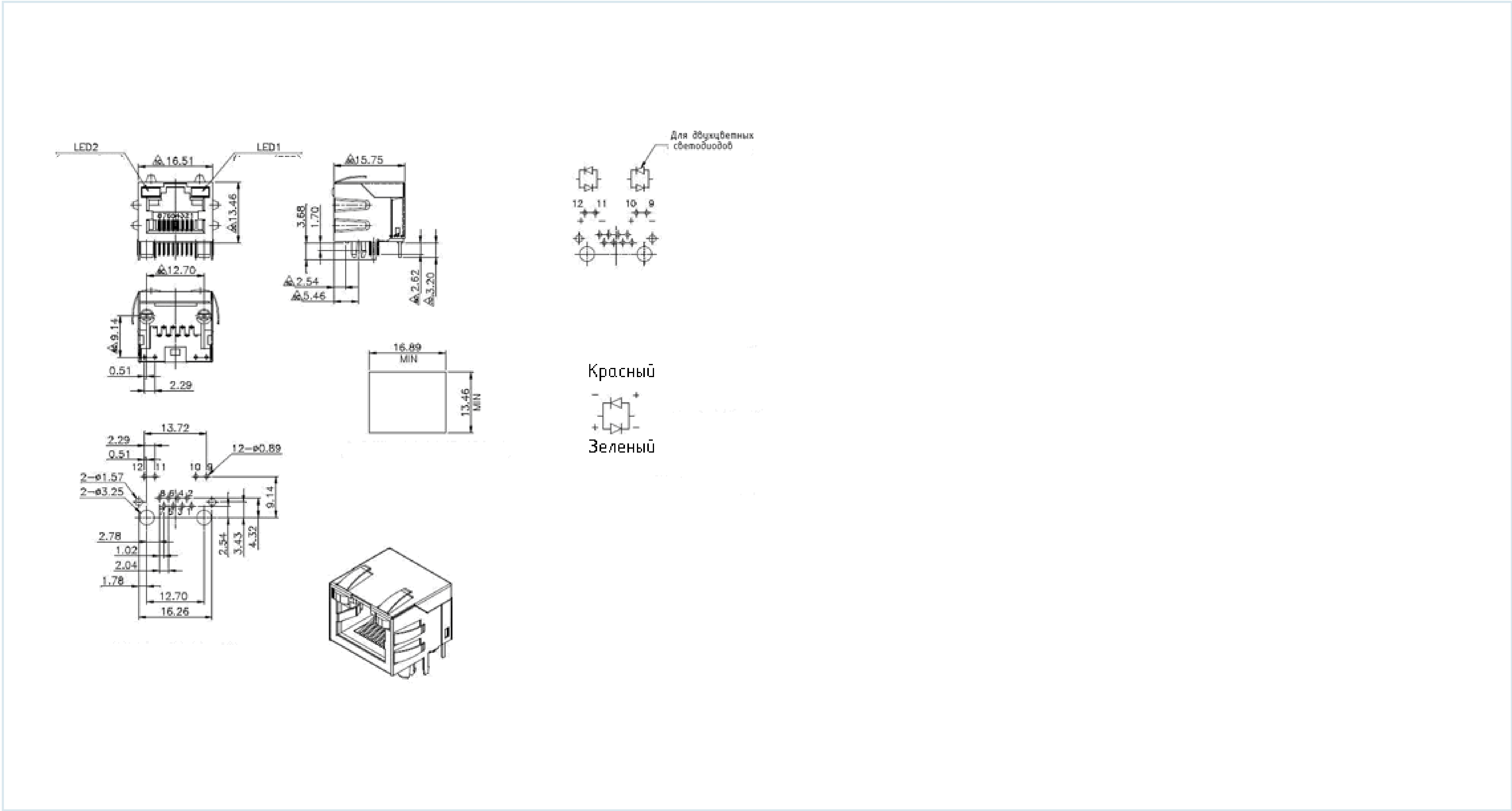
Схема изделия
