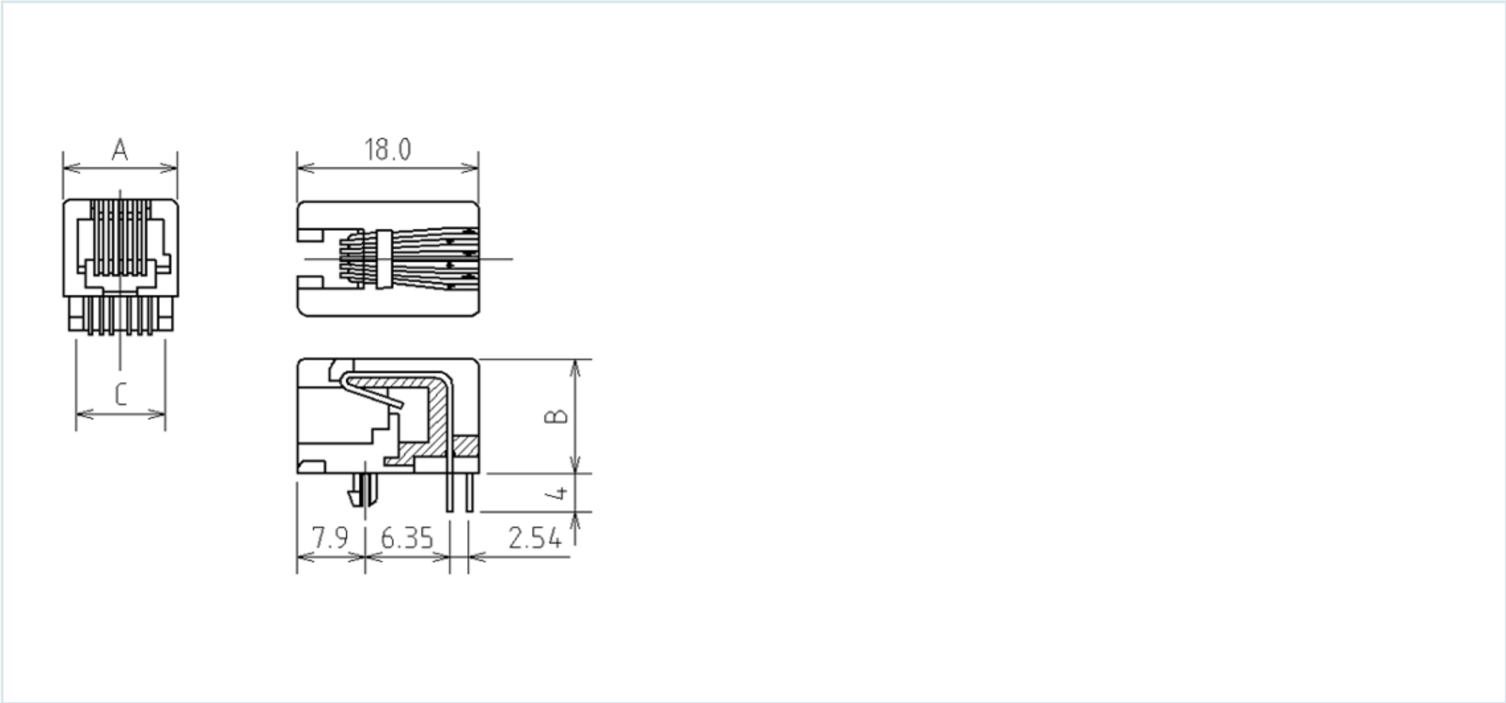
Схема изделия
