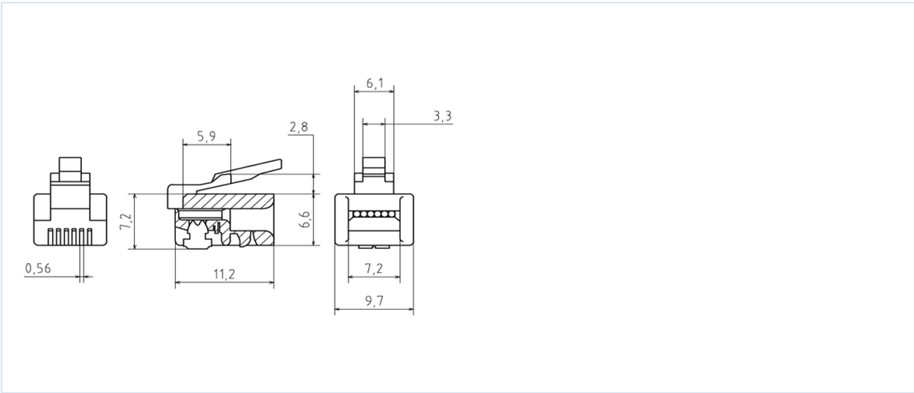
Схема изделия
