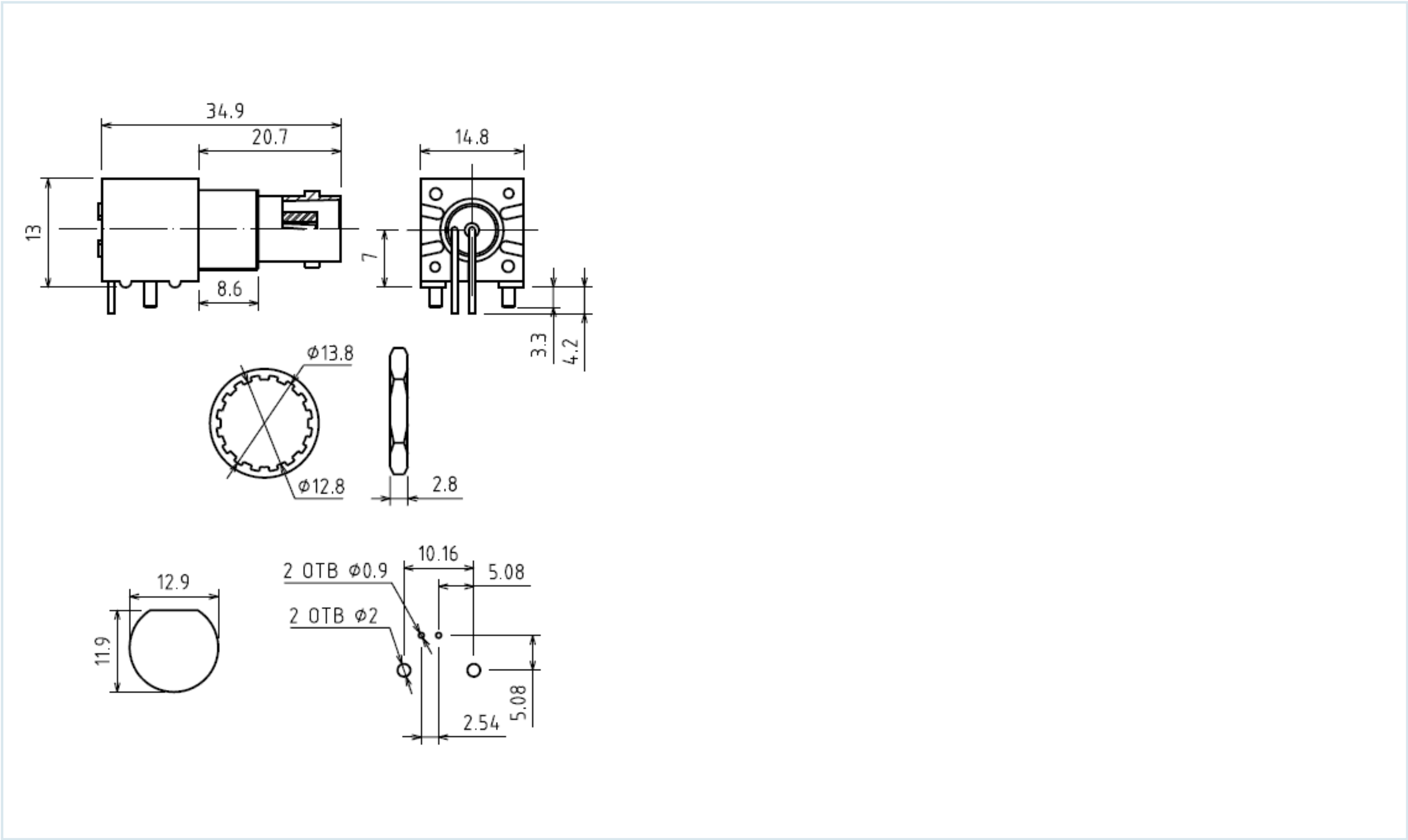
Схема изделия
