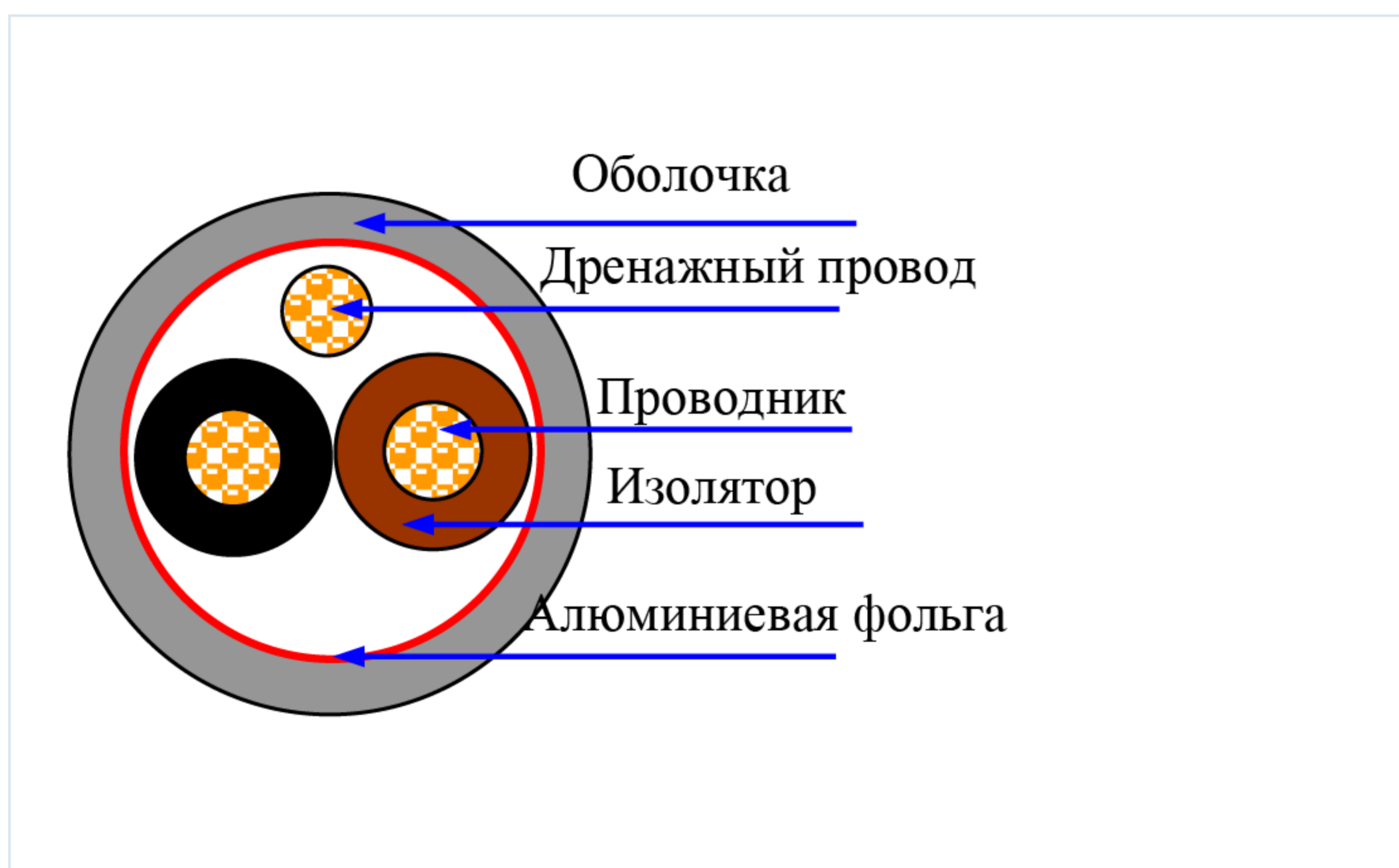
Схема изделия
