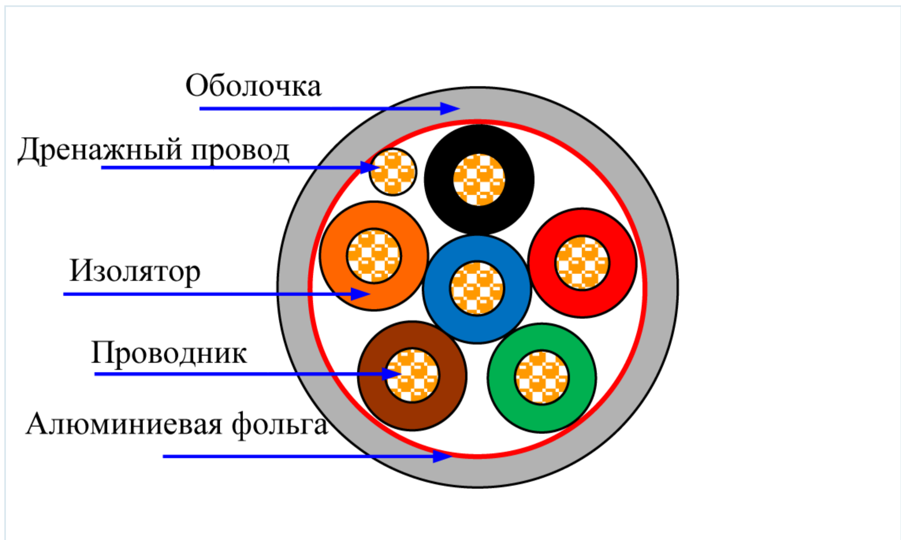
Схема изделия
