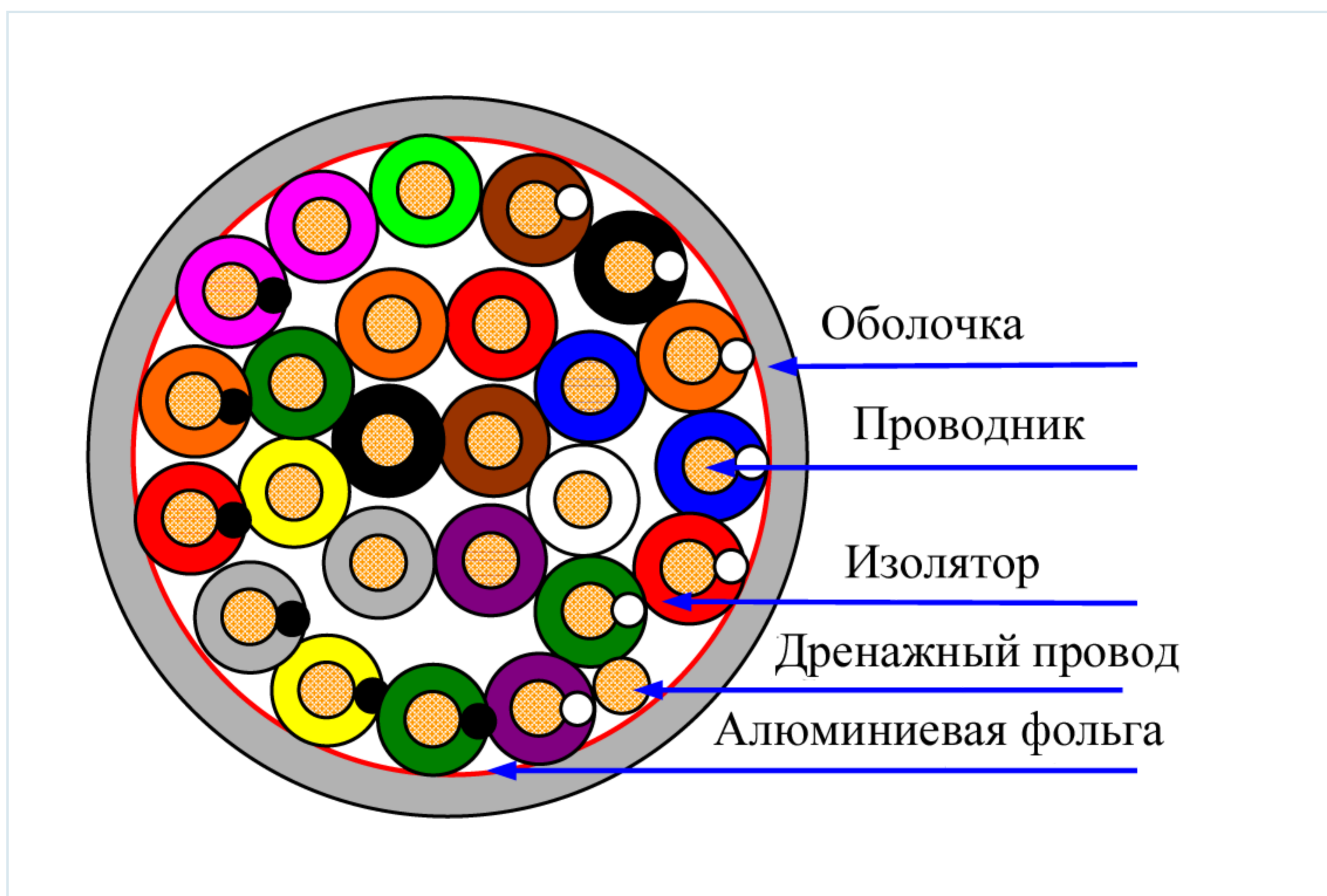
Схема изделия
