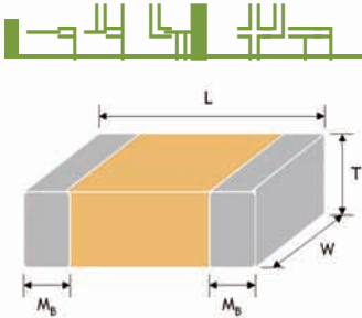
Рис. 1 контур MLCC
