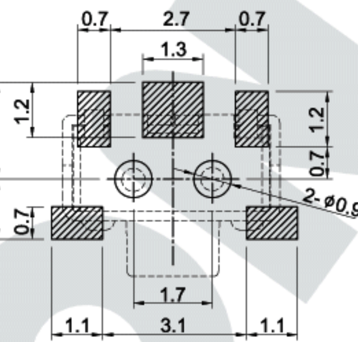
P.C.B. LAYOUT
