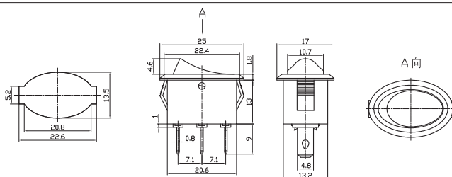
MIRS-101-10 ON-OFF 10A 125VAC;6A 250VAC SPST 3P
