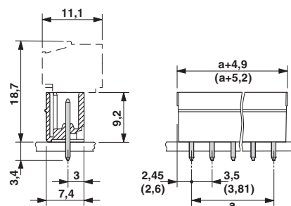
Чертеж
