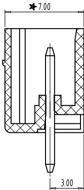
SECTION:A-A
