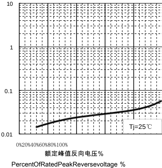
反向特性曲线 TypicalReverseCharacteristics
