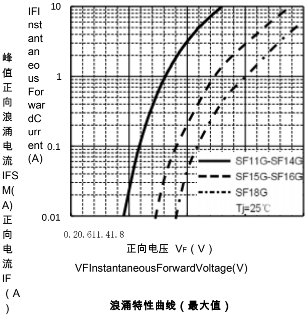
正向特性曲线 ( 典型值 ) TYPICALFORWARDCHARACTERISTIC
